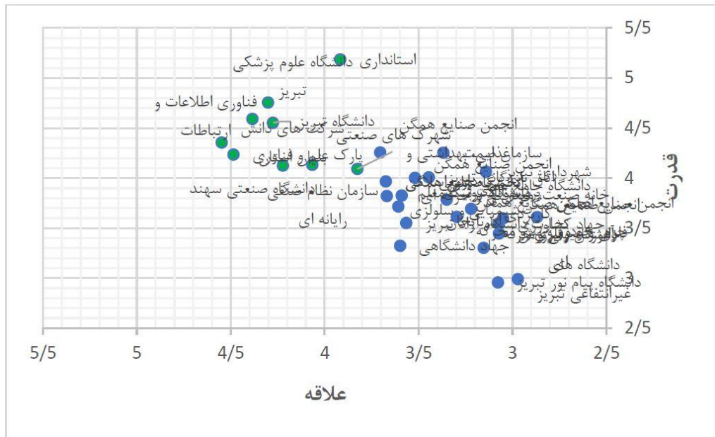
شکل ۲: ماتریس علاقه/قدرت
